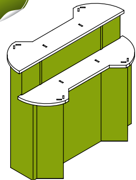
KIT MOSTRADOR DOBLE 1392x704x1200 mm. Mostrador a 900 y 1200 mm.
